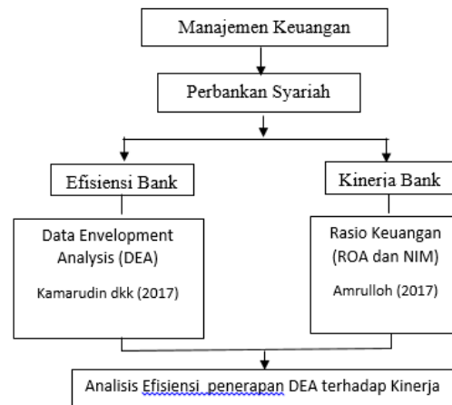
Gambar 2. Kerangka Penelitian
